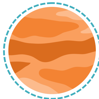
VENUS
