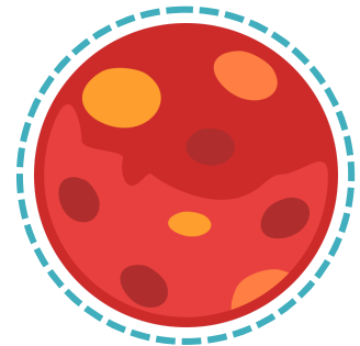
MARS
