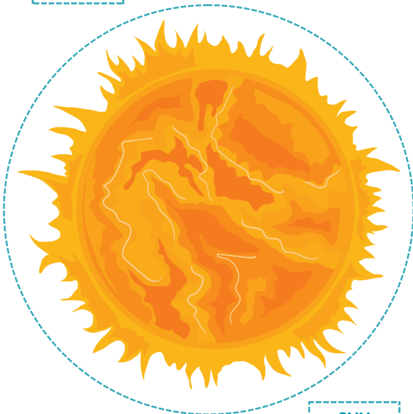
SUN
