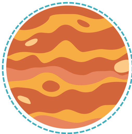
JUPITER
